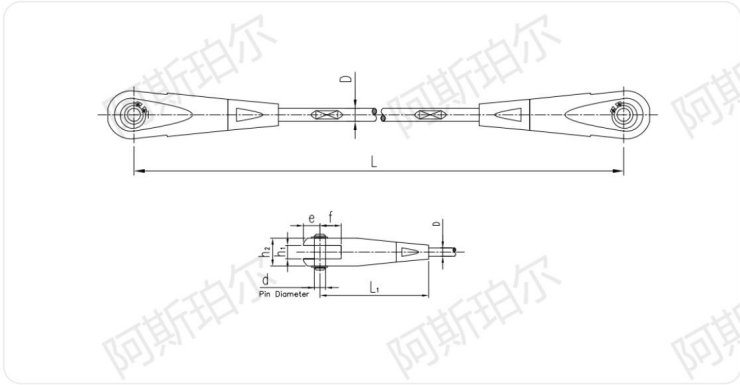
拉杆 / Tension Rod
