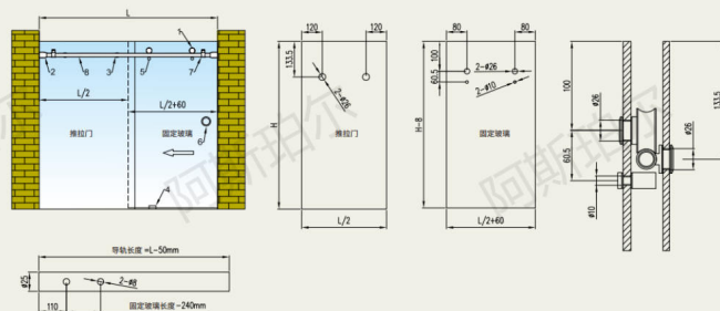
φ25 钢管(SSE02-B 系列) Illustration for φ25 pipe(SSE02-B Series)
